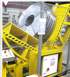
Mot. Kipptische 90° Mot. Upenders 90°
